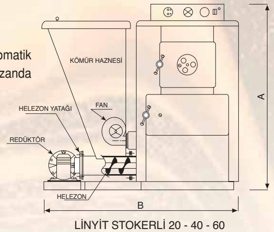
LİNYİTOMAT STOKERLİ 20 - 40 - 60
